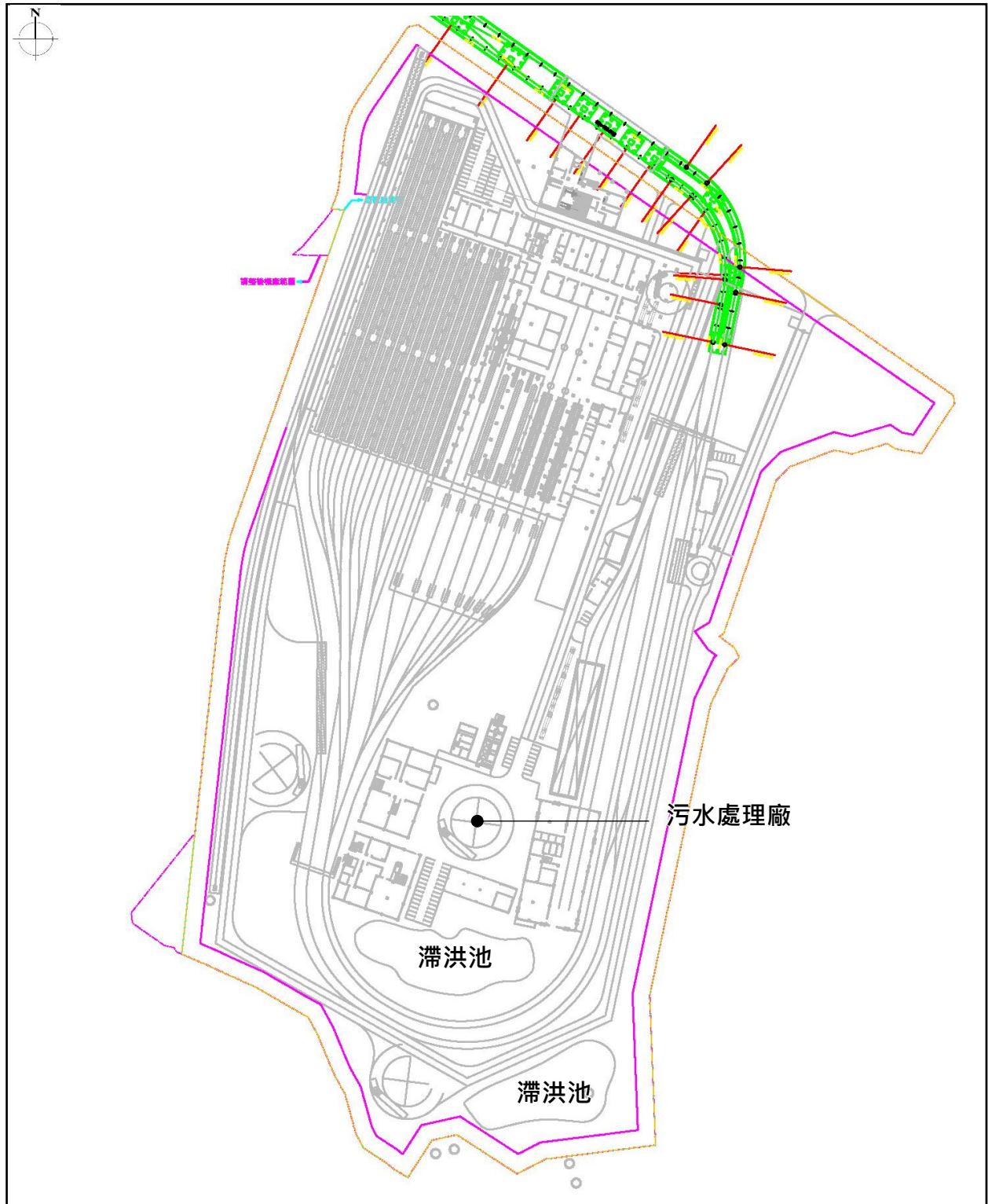
圖 4-4-1 高雄都會區大眾捷運系統黃線機廠配置示意圖
