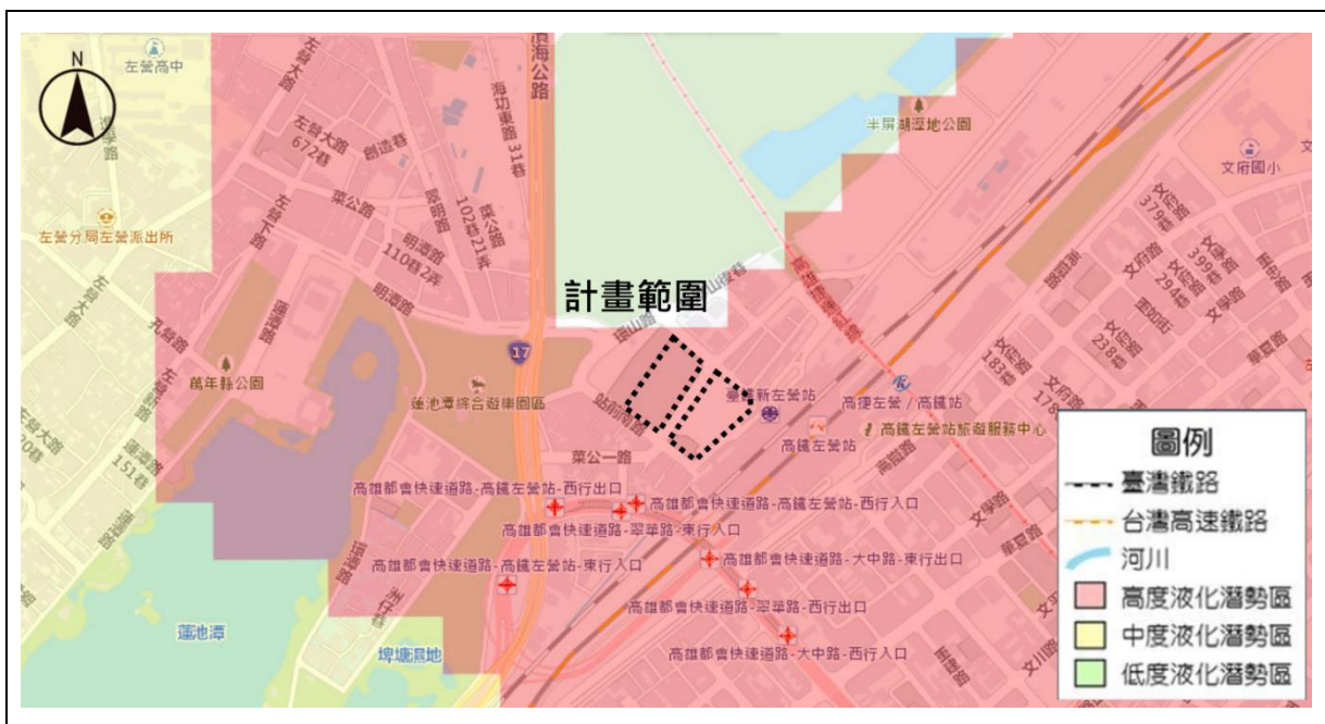
圖 16 本計畫及周邊地區土壤液化潛勢示意圖
