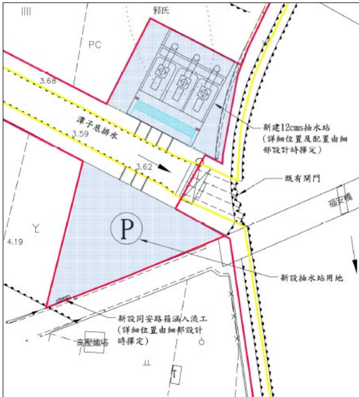
圖2 潭子底抽水站工程配置示意圖
