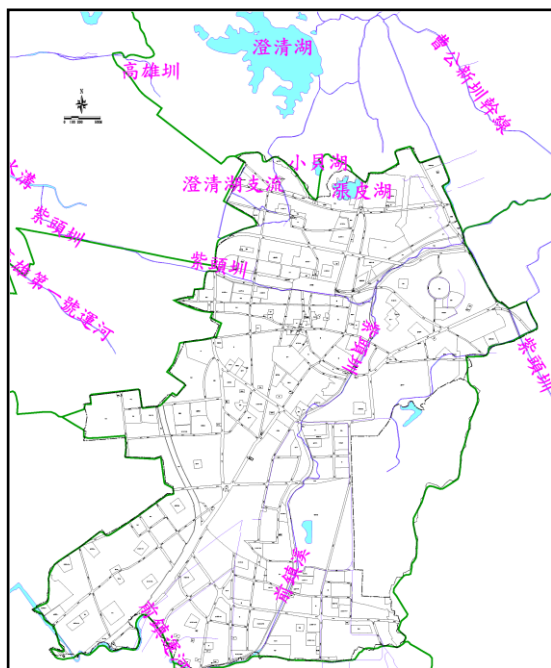
圖 3-1-4 水文系統分布示意圖
