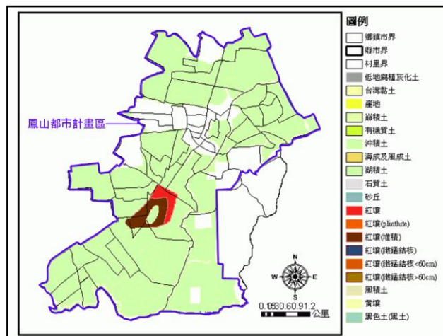
圖 3-1-2 土壤分布示意圖
