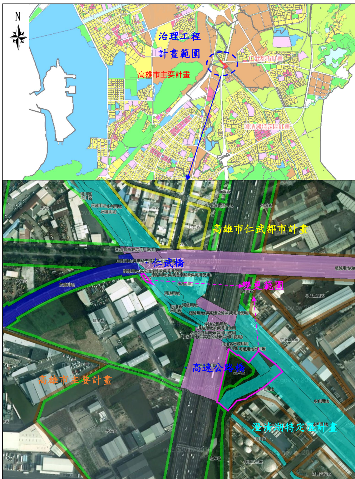
圖1 計畫位置示意圖
