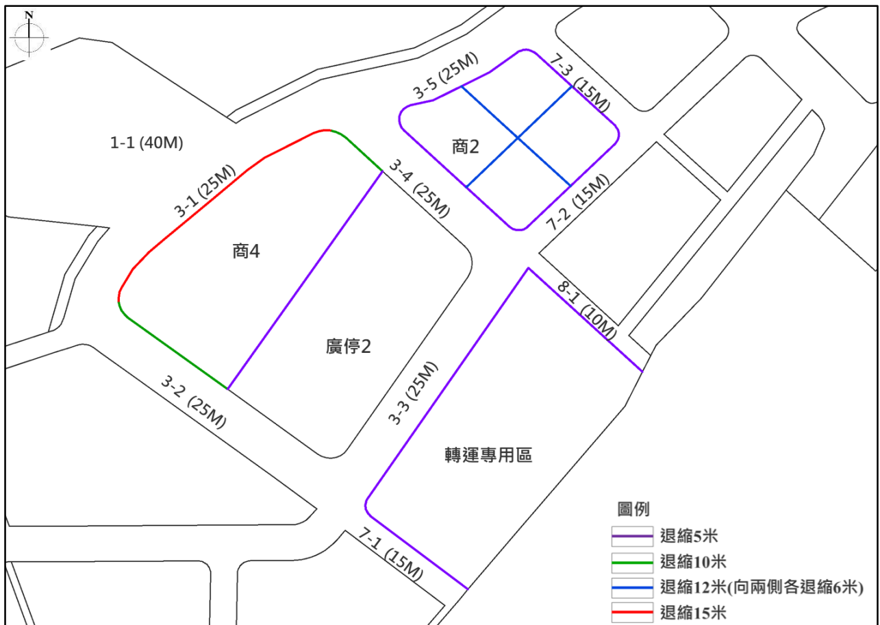
圖13 轉運專用區、第2種商業區、第4種商業區、廣場兼停車場用地退縮規定示意圖
