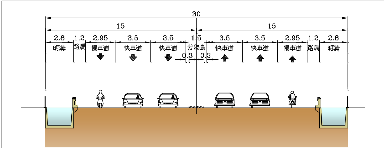
圖16 岡山區岡山北路、路竹區中山南路、中山路(巨輪興公司至路竹區國昌路、民強街口)現況配置示意圖
