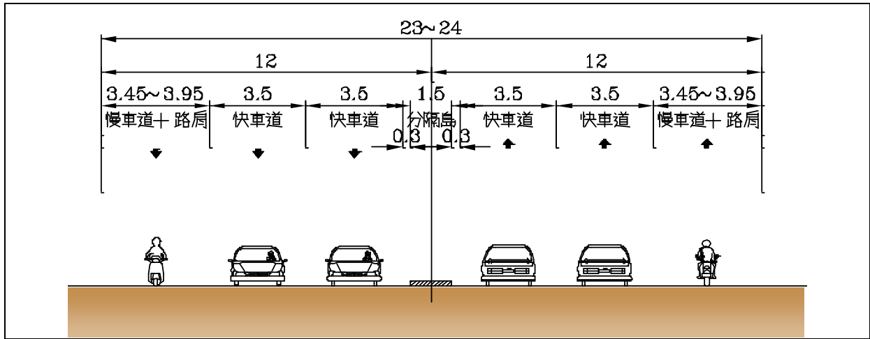
圖19 路竹區中山路(國昌路/民強街口至大仁路口北側)現況配置示意圖
