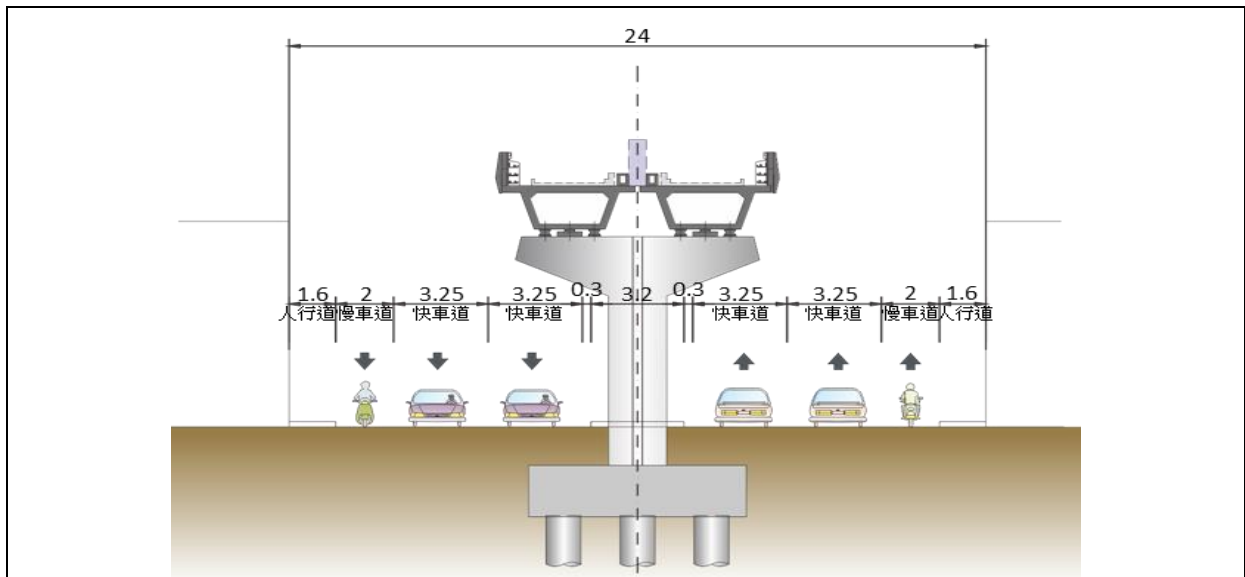
圖20 路竹區中山路(國昌路、民強街口至大仁路口北側)未來配置示意圖
