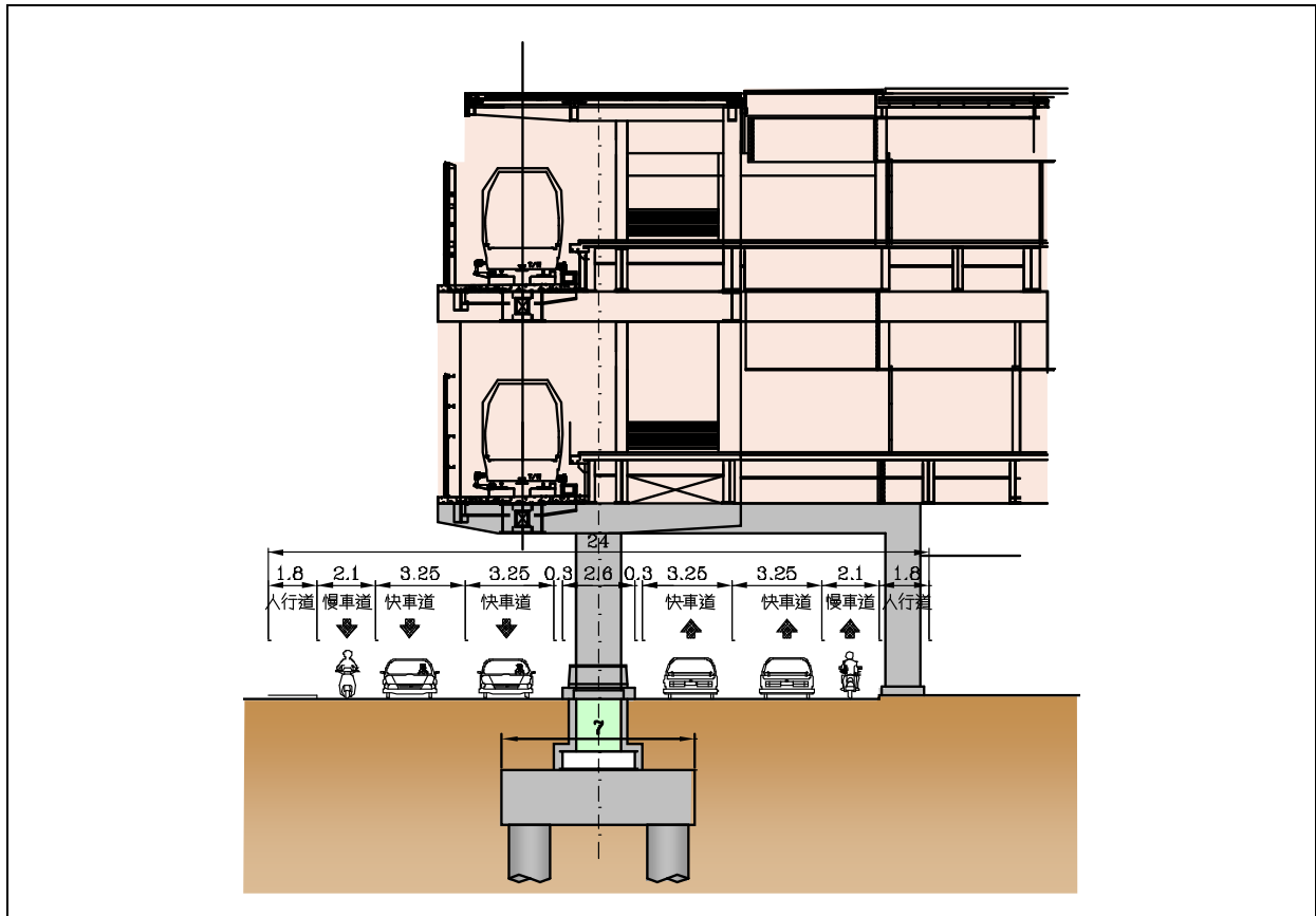
圖21 RK7 車站段未來車道配置示意圖
