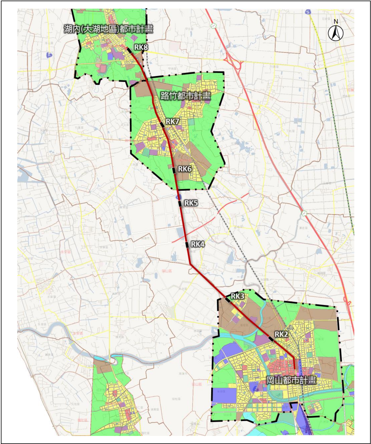
圖2 本計畫路線行經都市計畫情形示意圖
