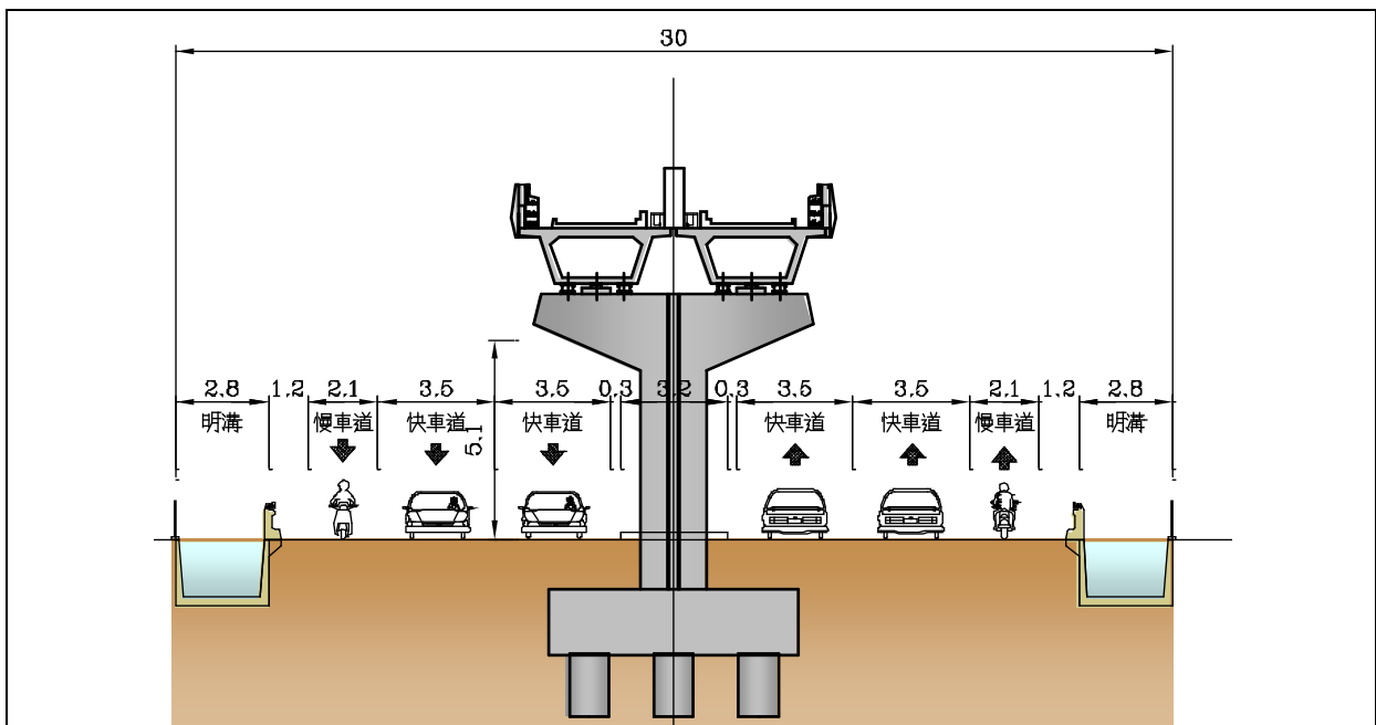
圖17 岡山區岡山北路、路竹區中山南路、中山路(巨輪興公司至路竹區國昌路、民強街口)未來配置示意圖
