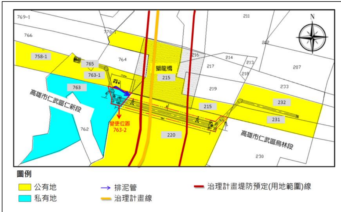
圖 7 獅龍溪水管橋工程地籍配置圖
