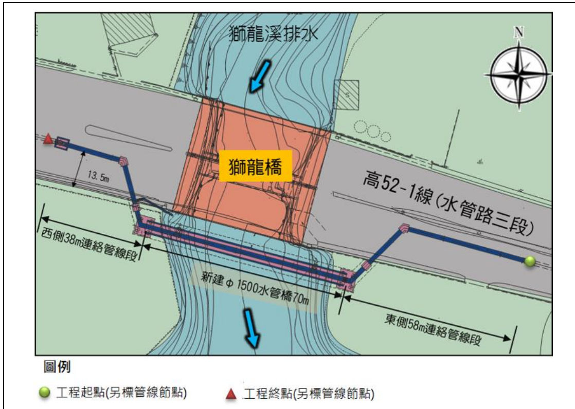
圖 6 獅龍溪水管橋工程位置示意圖
