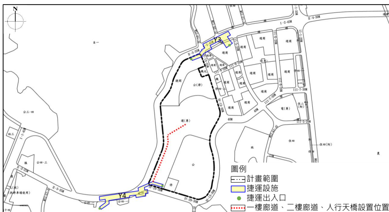
圖 6-7-1 一樓廊道、二樓廊道及人行天橋設置位置示意圖
